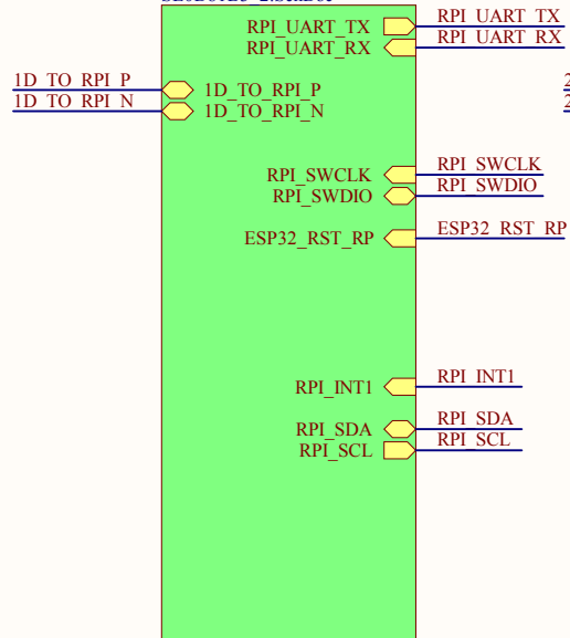
RP2040 SE0D81B3_2.SchDoc
